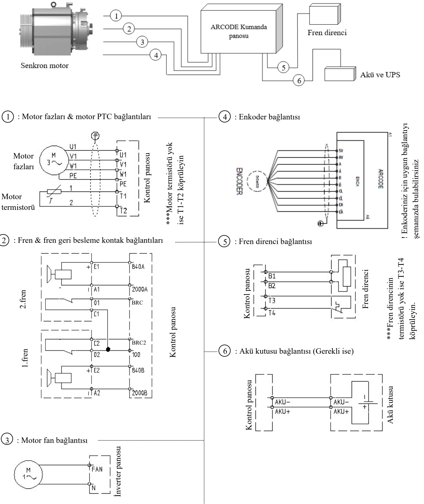
Şekil-4: Motor, fren, fan, enkoder, fren direnci ve akü bağlantıları
